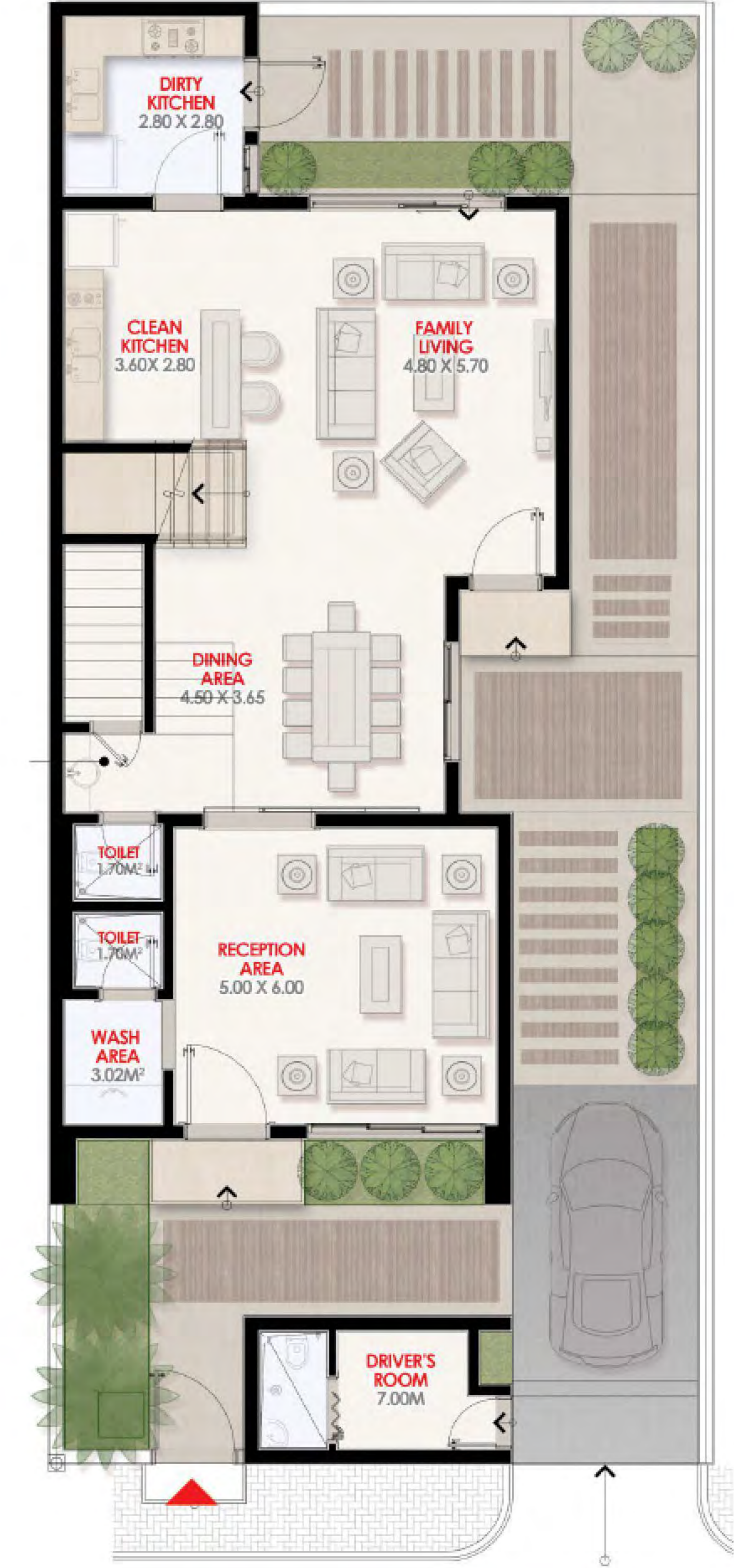
المسقط الأفقي للدور الأرضي
