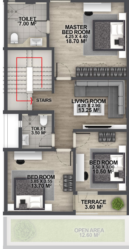
المسقط الأفقي للطابق الأول
